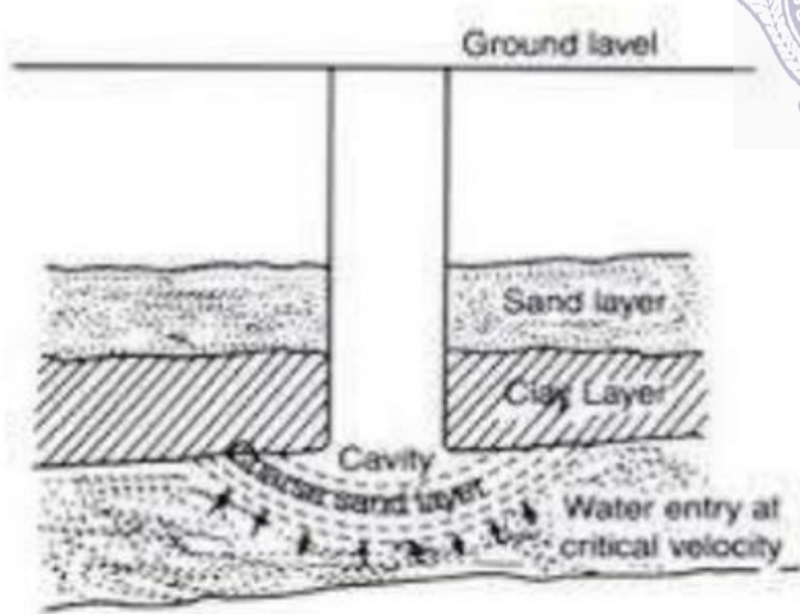
Fig. 18.2. Cavity type tubewell
