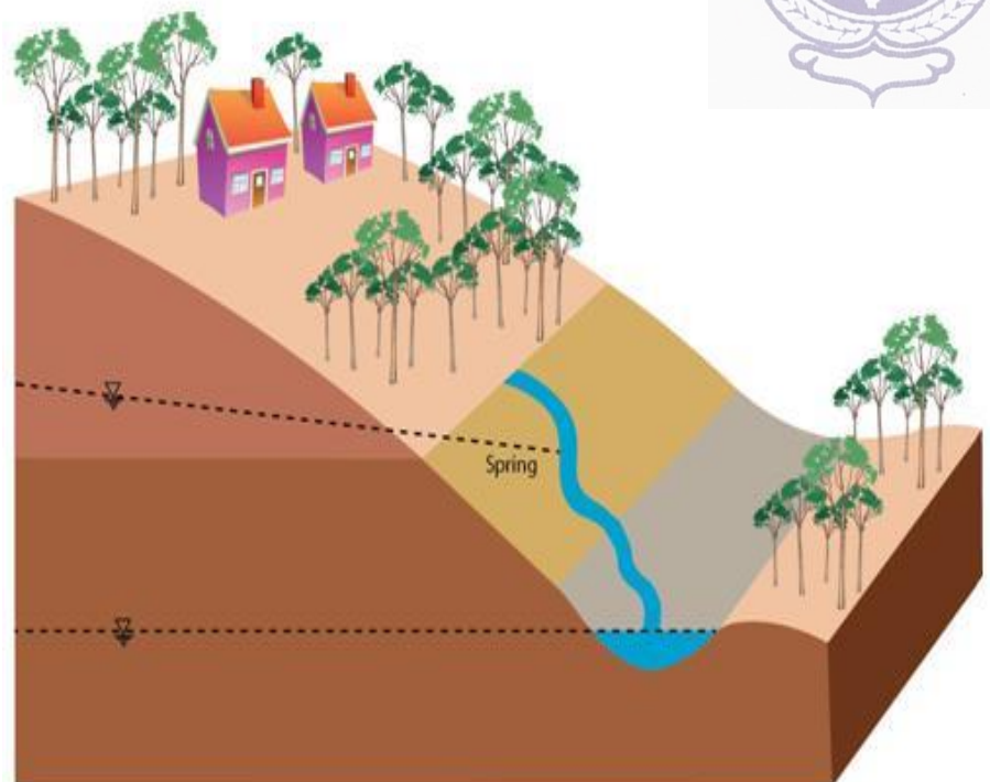
Fig. 2 Spring discharge
